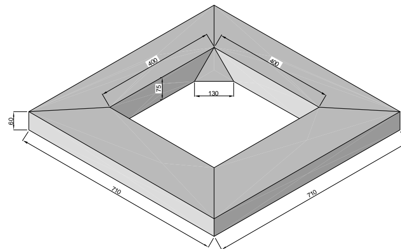
28" x 28" Chimney Cap
