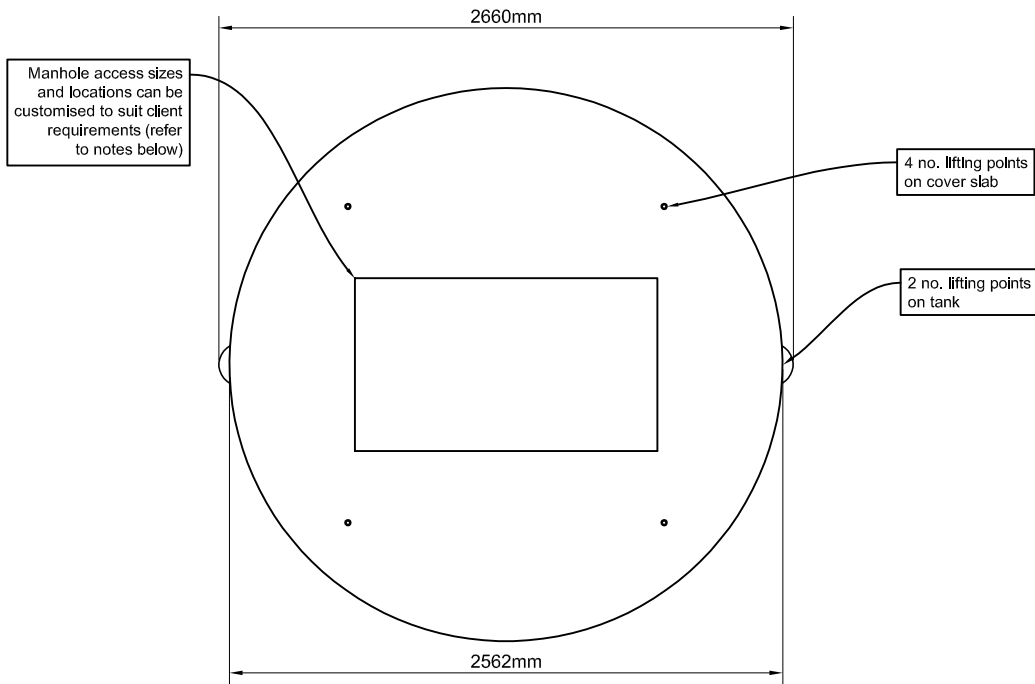
LID PLAN
